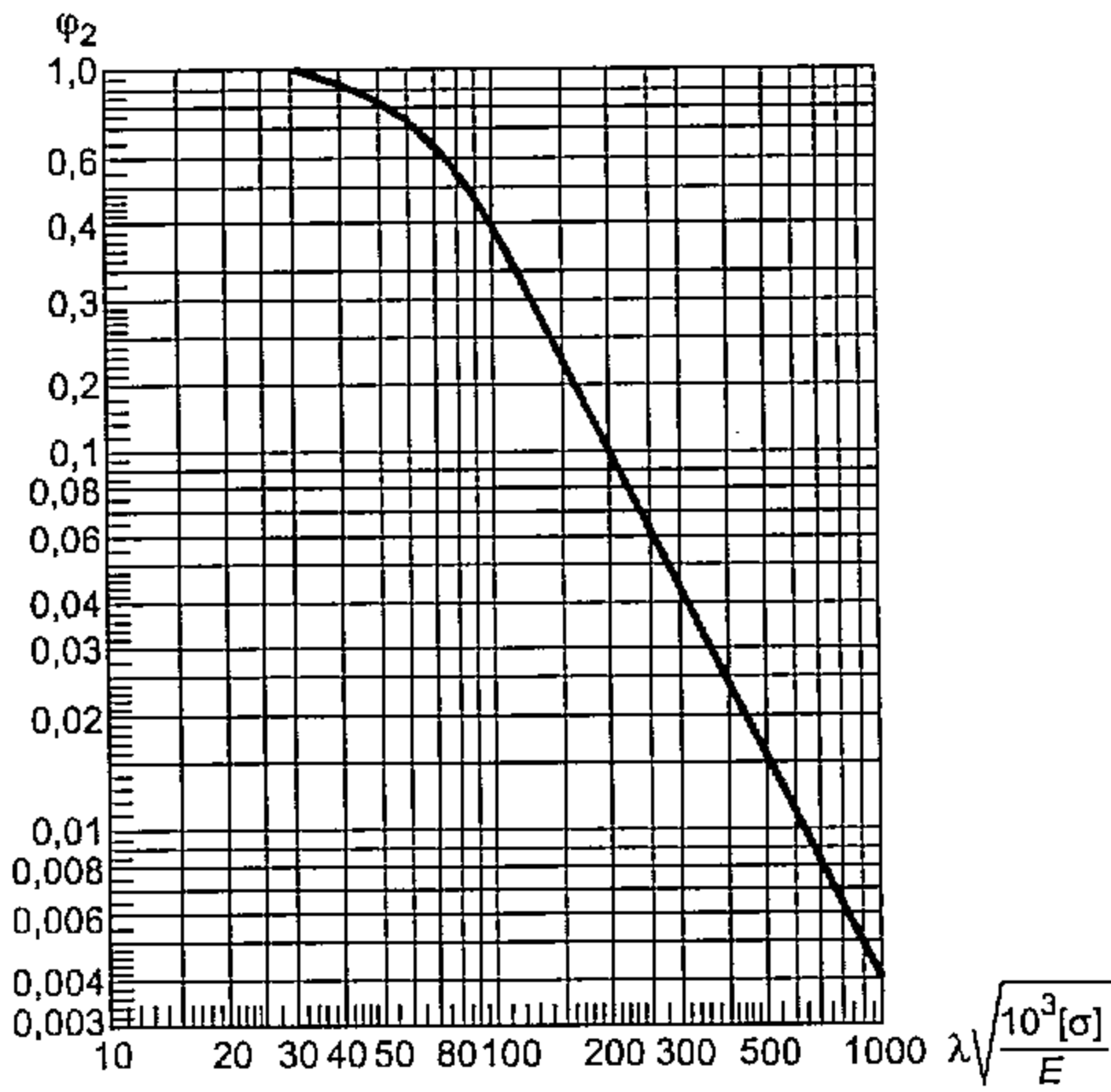
Рисунок 6 — График для определения коэффициента \varphi_2
